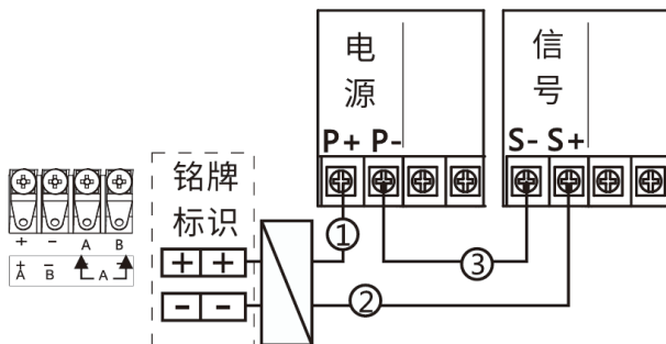
图 23 本安型两线制 4 ~ 20mA
