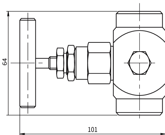
图 14 截止阀 - 输入端 1/2NPT 内螺纹，输出端 1/2NPT 内螺纹
