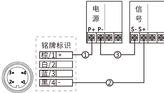
图 24 两线制 4 ~ 20mA 带航插头
