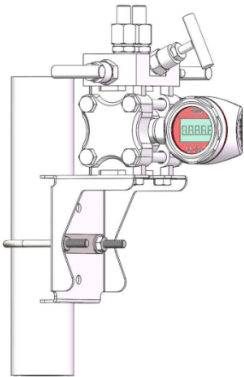
图 11 管装弯支架
