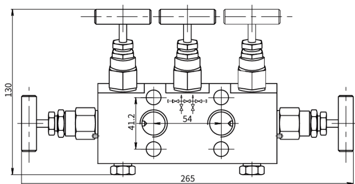
图 20 五阀组 - 中心距 54mm
