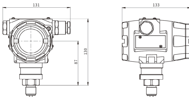
带显示整机尺寸图
