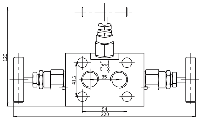
图 18 三阀组 - 中心距 35mm
