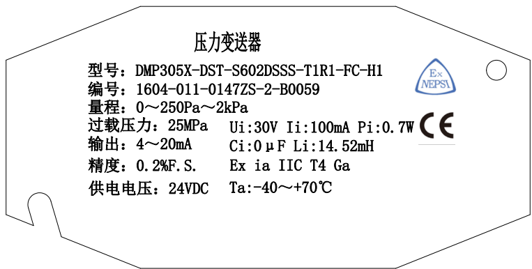
图 1 铭牌
