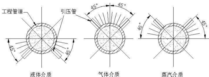
图 21 引压口位置
