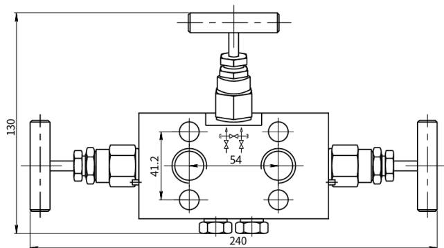
图 19 三阀组 - 中心距 54mm
