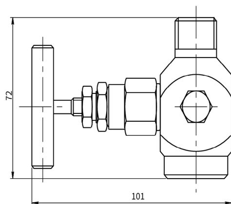
图 15 截止阀 - 输入端 1/2NPT 内螺纹, 输出端 1/2NPT 外螺纹
