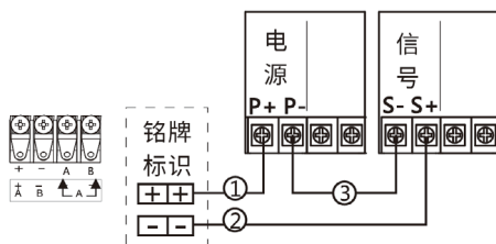
图 22 两线制 4 ~ 20mA
