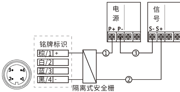
图 25 两线制 4 ~ 20mA 带航插头
