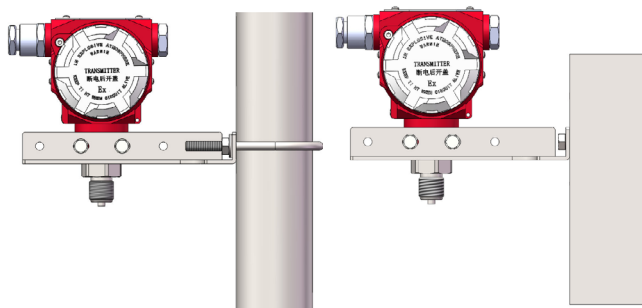
图 3 支架安装
