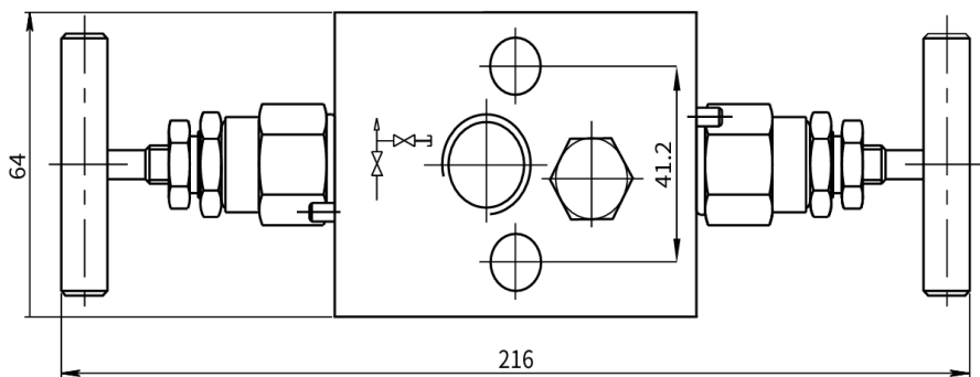
图 17 共面二阀组
