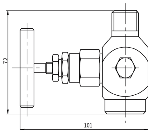
图 16 截止阀 - 输入端 1/2NPT 外螺纹, 输出端 1/2NPT 外螺纹
