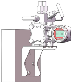
图 12 板装弯支架
