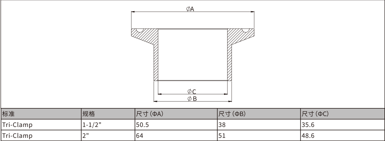
焊接转接件 (Z1-Z1) (单位:mm)
