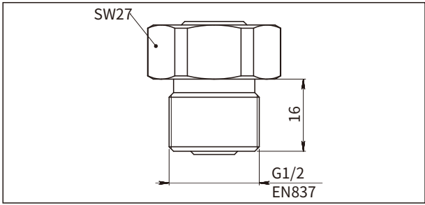
过程连接 (K01-K02) (单位:mm)
