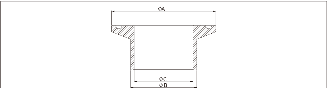
焊接转接件 (Z1-Z2) (单位:mm)
