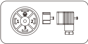
DIN43650 (D1)
