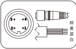
航插直头 (J4)
