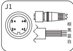
M12*1-4芯航空插头 (H1)、航插直头 (J1)、航插弯头 (J2)、航插直头 (J4)、航插弯头 (J5)
